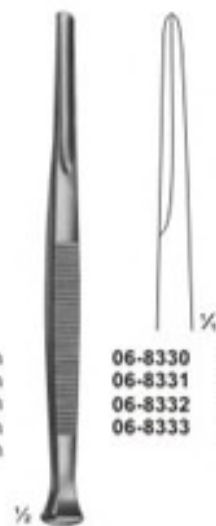
PARTSCH 06-8330 - 06-8333 Gouges 140 mm
