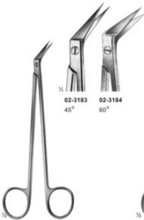
02-3183 - 02-3184 DE BAKHEY Size: 155 mm
